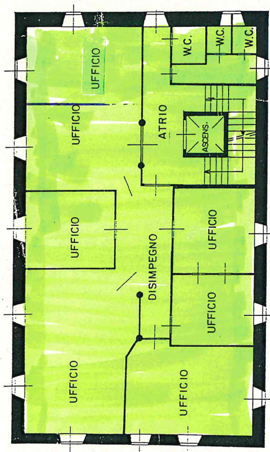
PRIMO PIANO — H = 2.60
